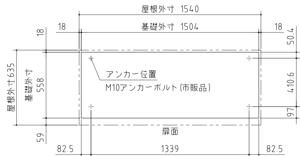
ベタ基礎図
