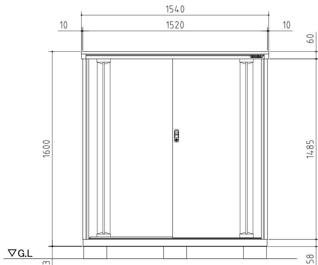
正面図
