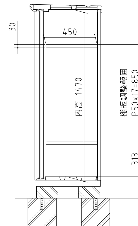
断面図
